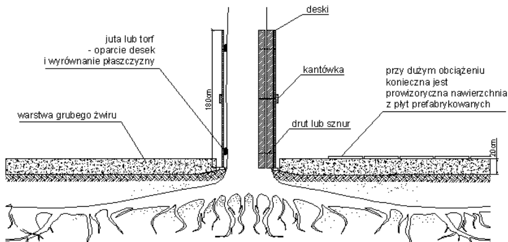
Rys. 1. Zabezpieczenie drzewa na czas budowy
