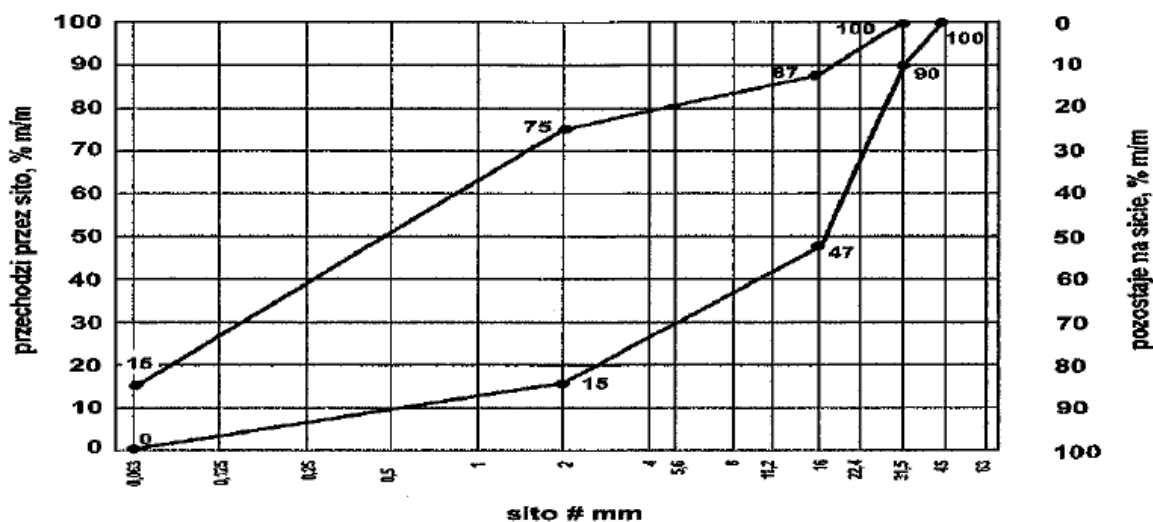
Rysunek 1. Mieszanka niezwiązana 0/31,5 do warstwy ulepszanego podłoża stabilizowanego georusztem lub układanej na geotkaninie
